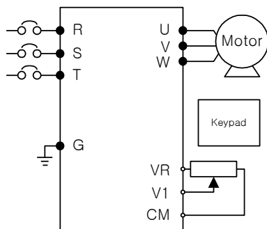
Câblages
