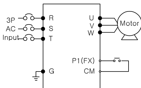
Câblages
