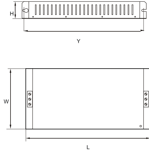
Filtres Standard
