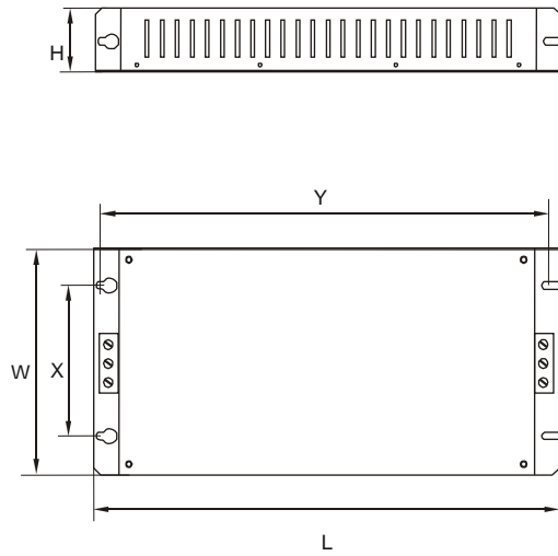
Filtres FFM (Footprint)
